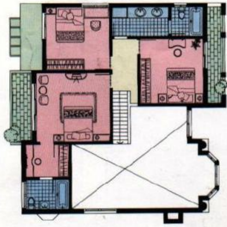
二樓平面圖 2nd Floor Plan
